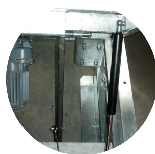
Molla a gas per facilitare l'apertura della pedana
